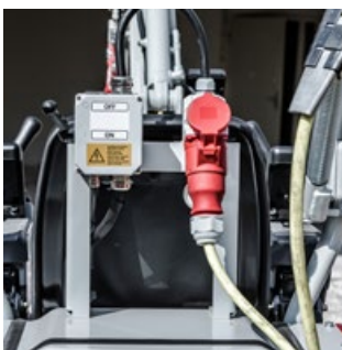
Schakelaar diesel/elektrisch
