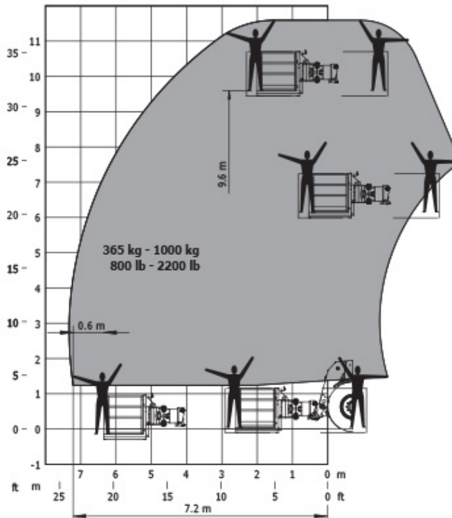
Machine op banden met platform
